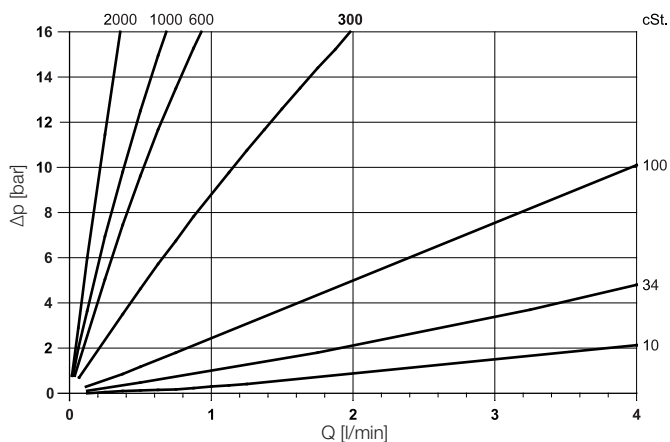
SCVF-004 \Delta p - Viskosität
