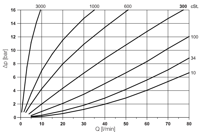
SCVF-040/060/080 \Delta p - Viskosität
