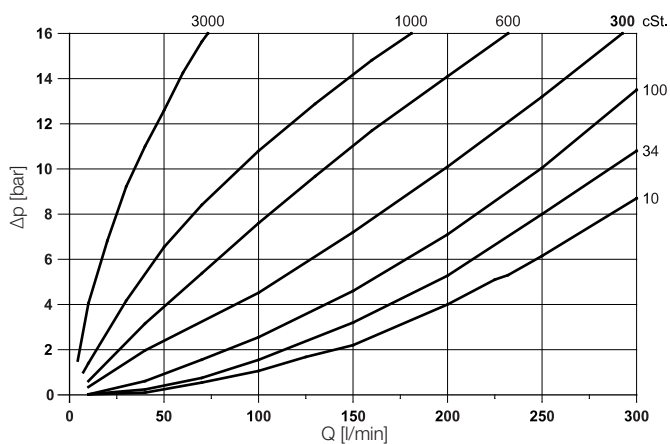
SCVF-300 \Delta p - Viskosität
