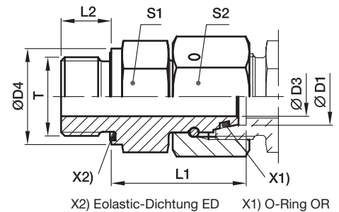
X2) Eolastic-Dichtung ED X1) O-Ring OR
