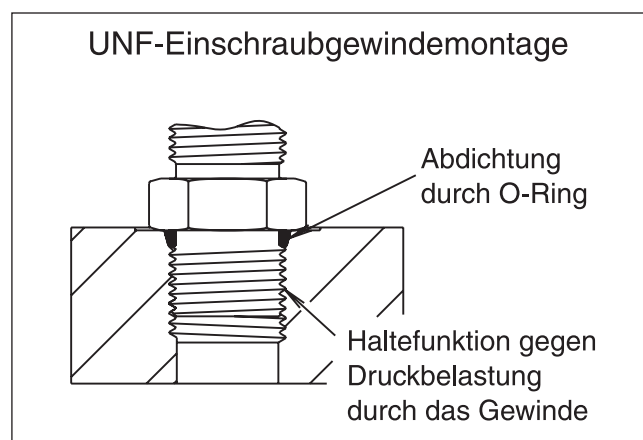
Abb. 6 – UNF-Einschraubgewindemontage
