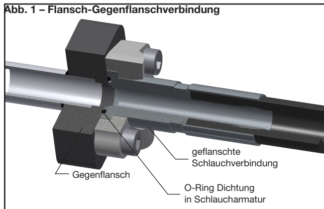
Abb. 1 – Flansch-Gegenflanschverbindung
