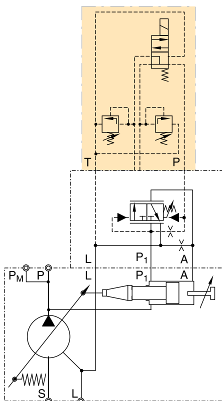
Schaltplan PVAC2P*
