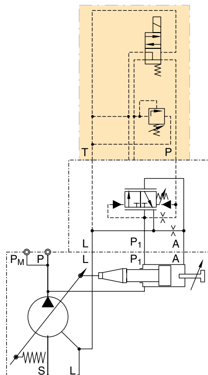
Schaltplan PVAC1E*
